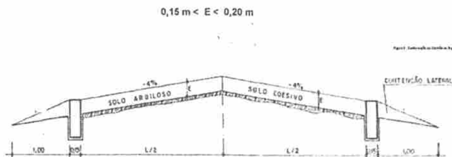
Figura 5 - Conformação do colchão de areia
