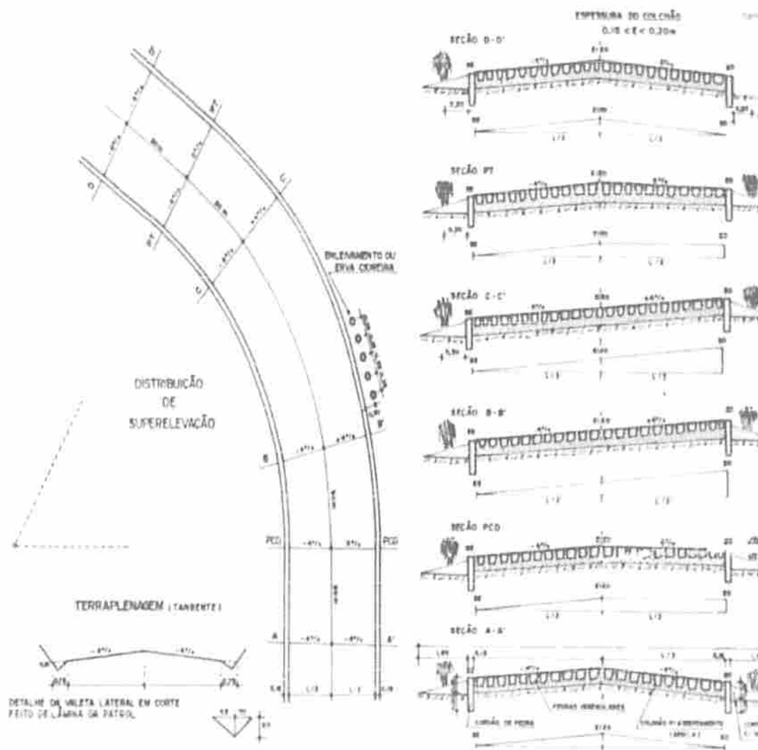
Figura 3 - Superelevação - Curva para Esquerda
