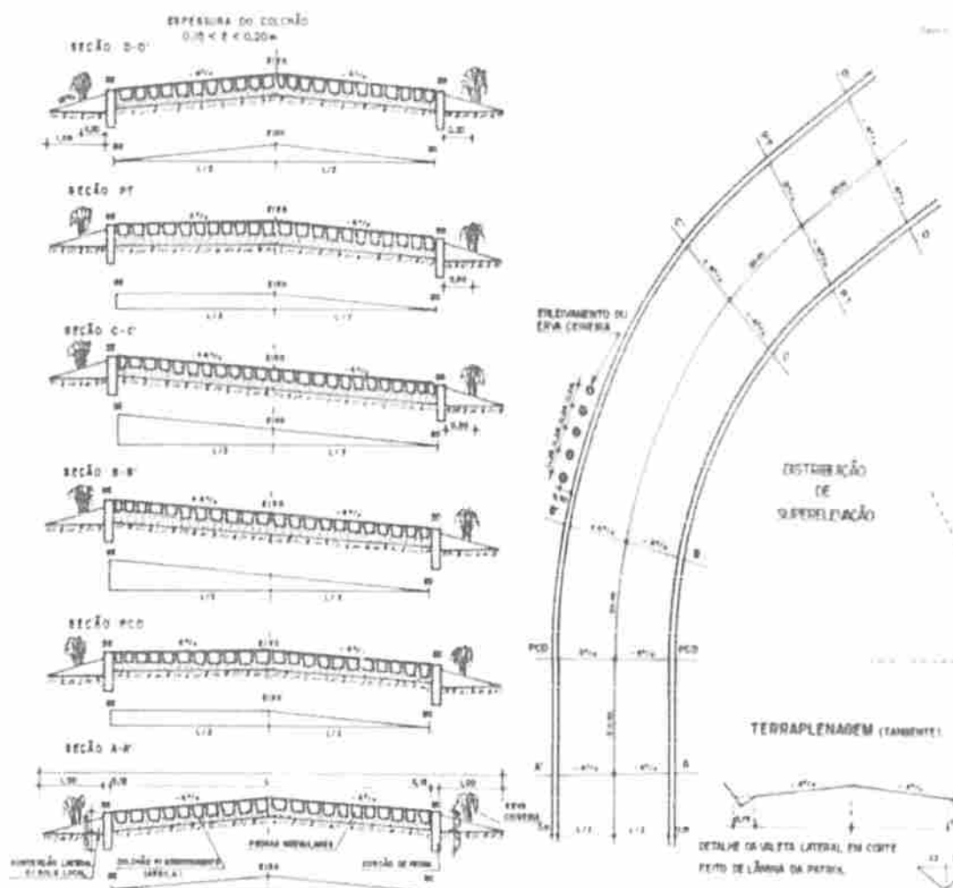
Figura 2 - Superelevação - Curva para a Direita
